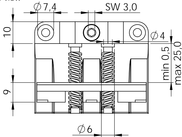
Seitenansicht von links side view left
