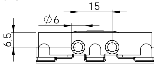
Vorderansicht front view
