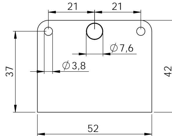
Untersicht bottom view
