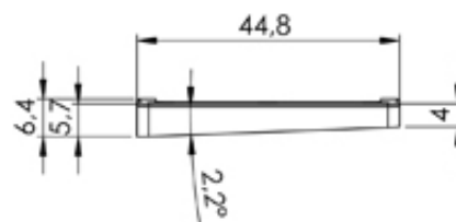
Seitenansicht von links side view left
