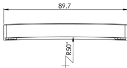
Draufsicht top view
