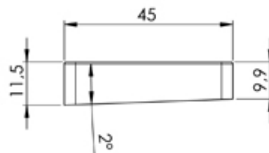
Seitenansicht von links side view left
