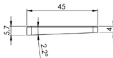
Seitenansicht von links side view left
