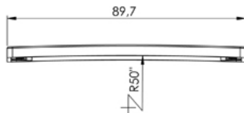
Draufsicht top view
