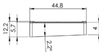
Seitenansicht von links side view left
