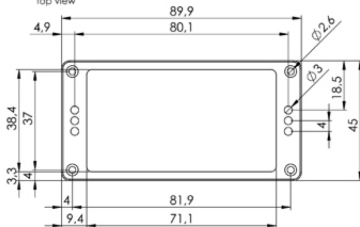
Draufsicht top view
