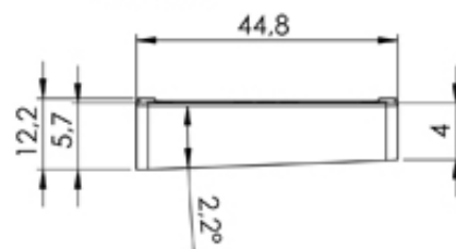
Seitenansicht von links side view left
