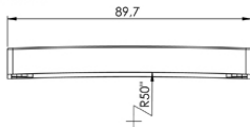
Vorderansicht front view
