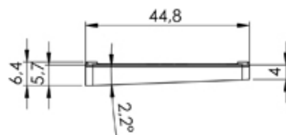
Seitenansicht von links side view left
