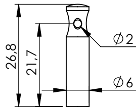
Locking 19,5 1002XXXX.XX.52
