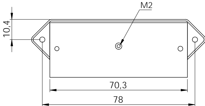
Untersicht bottom view
