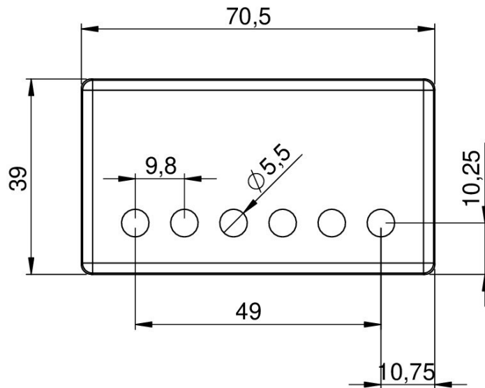
Draufsicht top view
