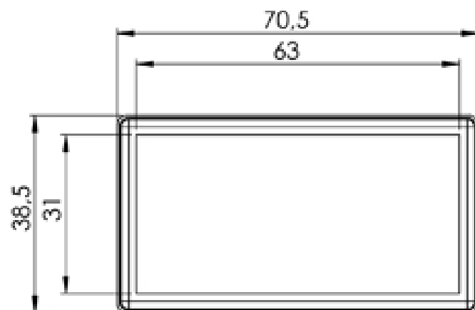
Draufsicht top view
