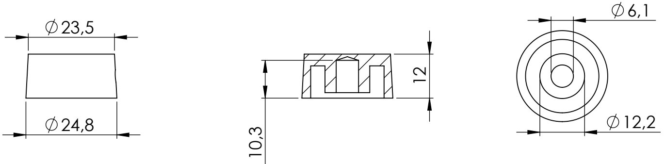
Kegelstumpf frustum PK: 1503XXXX
