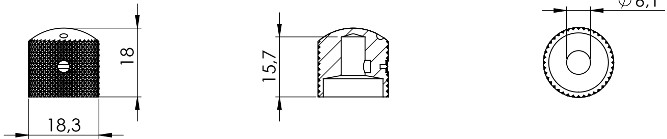
Zylinder cylinder PK: 1502XXXX
