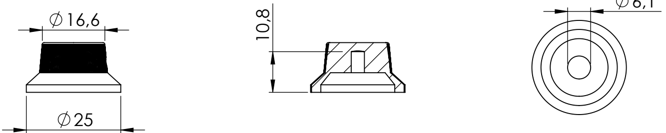
Hutform hat shape PK: 1501XXXX
