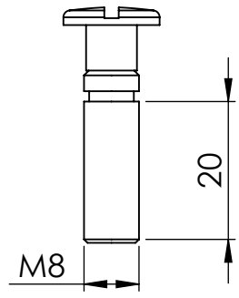
Höhenverstellerschraube Studs
