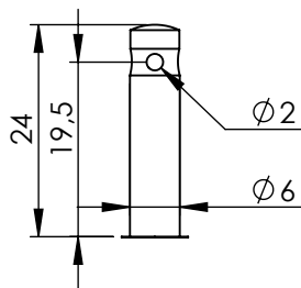
Locking 19,5 1004XXXX.XX.52
