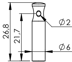
Locking 19,5 1004XXXX.XX.52
