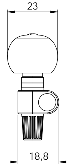
Rückansicht back view
