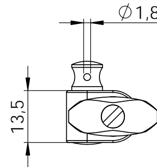
Seitenansicht von links side view left
