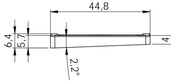
Seitenansicht von links side view left
