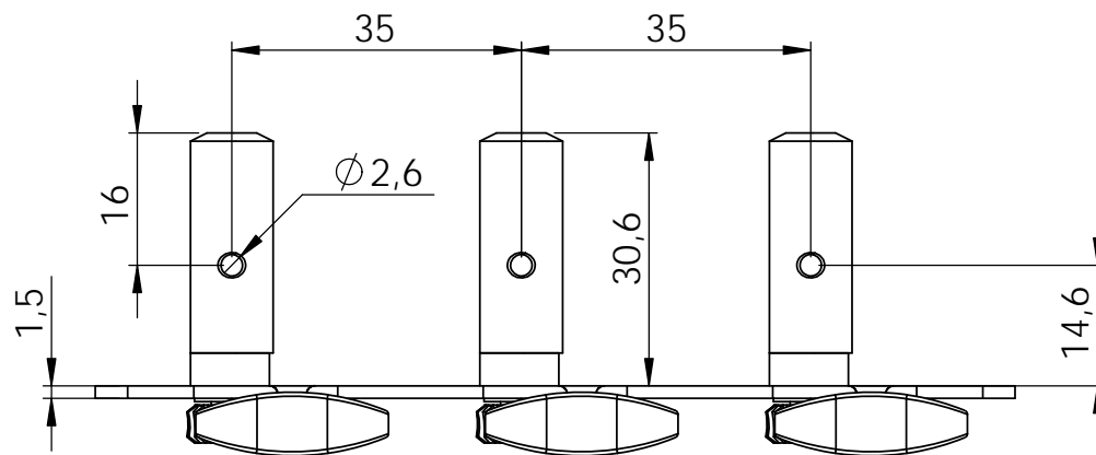
Draufsicht top view
