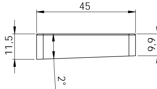
Seitenansicht von links side view left
