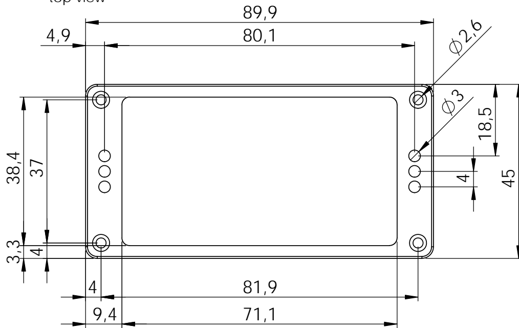
Draufsicht top view
