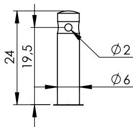
Locking 19,5 1056XXXX.XX.52
