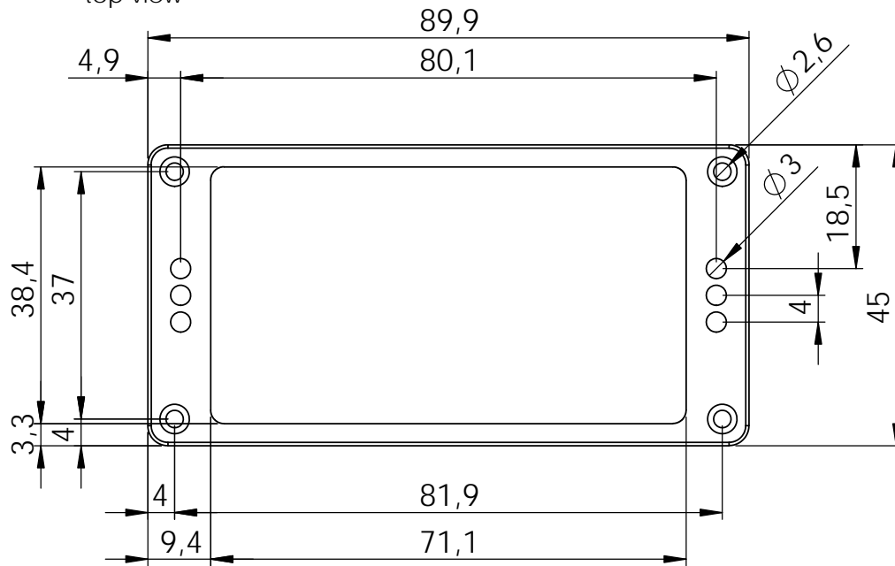
Draufsicht top view
