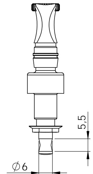
Seitenansicht von rechts side view right
