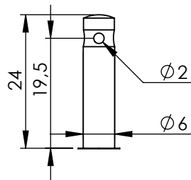
Locking 19,5 1002XXXX.XX.52
